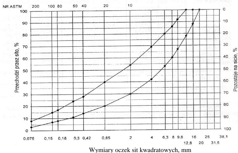
Rys. 7. Krzywe graniczne uziarnienia mieszanki mineralnej BA od 0 do 16 mm do warstwy wyrównawczej, wiążącej i wzmacniającej nawierzchni drogi o obciążeniu ruchem od KR1 do KR2
